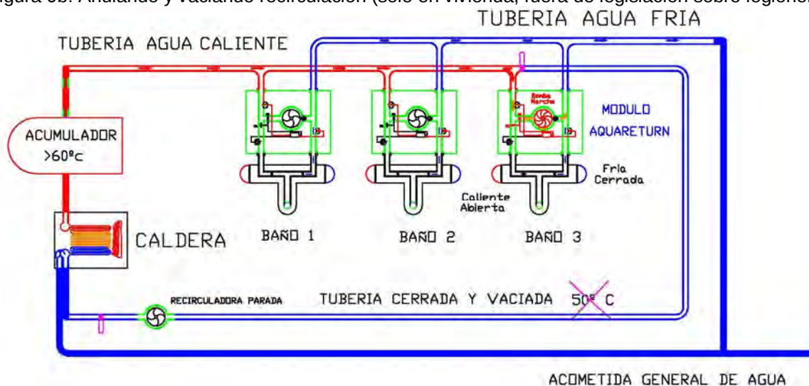
Figura 9b: Anulando y vaciando recirculación (sólo en vivienda, fuera de legislación sobre legionella).
