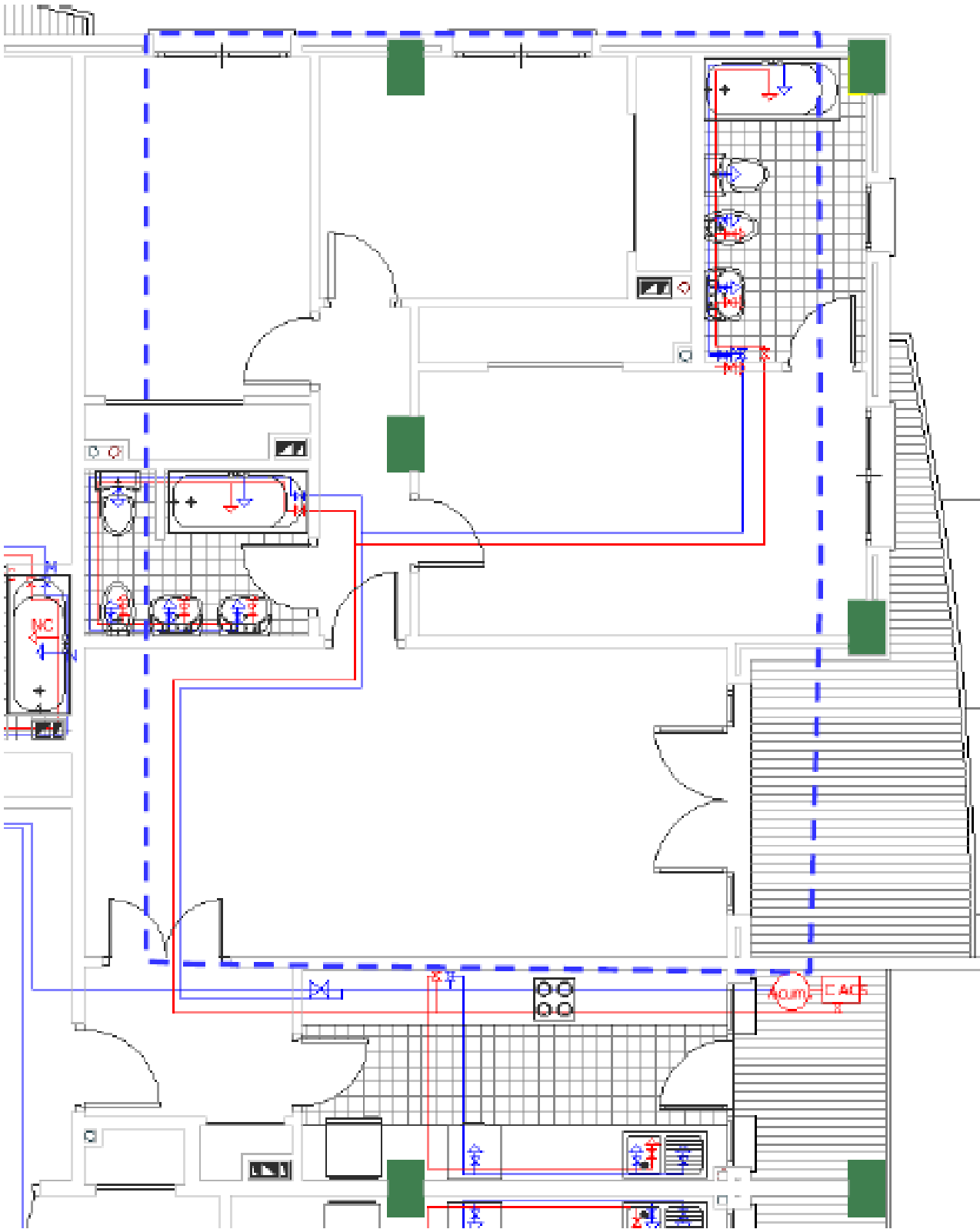
Figura 8: Vivienda tipo utilizada en simulaciones de volúmenes de ACS no aprovechados (ITA-UPV).
