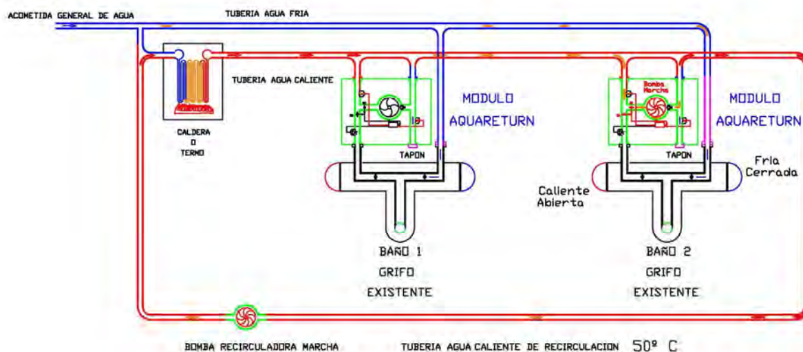
Figura 10: Esquema de funcionamiento para prevención de legionella (sin acumulador de ACS).
